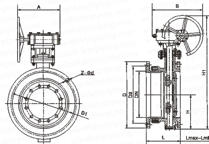
主要连接尺寸 Main Connection Dimension
