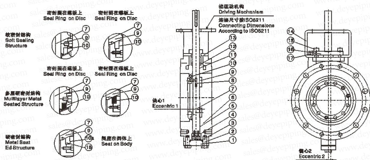
主要连接尺寸 Main Connection Dimensions
