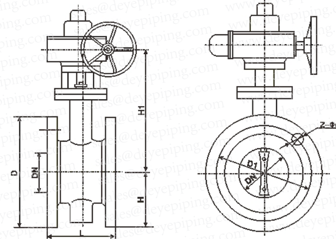
主要连接尺寸 Main connection dimensions 单位Unit:mm
