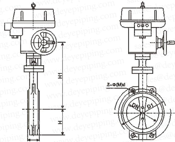
主要连接尺寸 Main Connection Dimensions 单位Unit:mm
