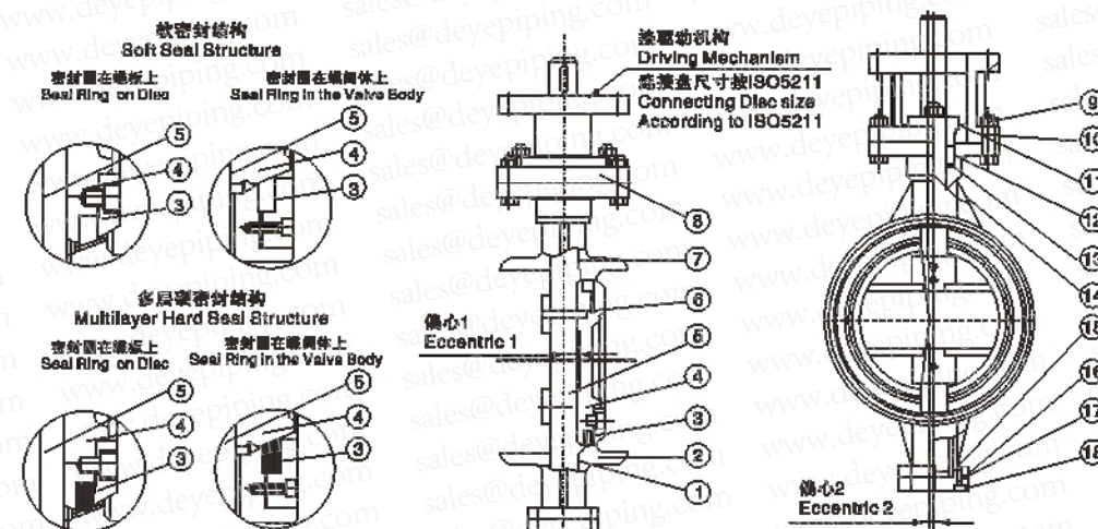
主要连接尺寸 Main Connection Dimensions
