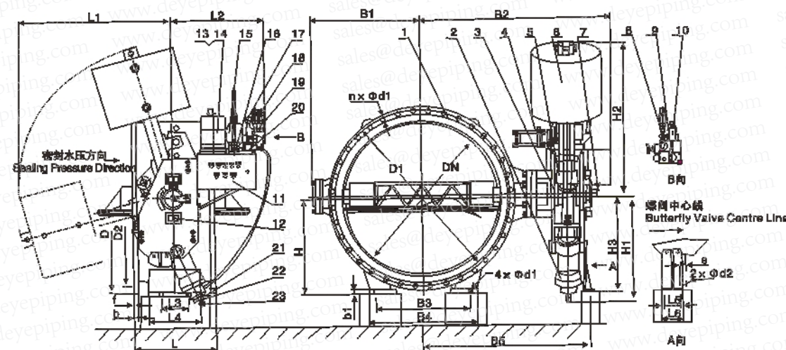
1、阀体 2、油缸 3、传动支架 4、摇臂 5、杠杆 6、重锤 7、开度电位器 8、常开截止阀 9、常闭截止阀 10、电磁阀 11、压力开关 12、行程开关 13、电机 14、油泵 15、蓄能器 16、手动泵 17、压力表 18、流量控制阀 19、溢流阀 20、电气控制箱 21、快关调节阀 22、慢关调节阀 23、快慢角度调节 1、Body 2、Hydrocylinder 3、Transmission Bracket 4、Rocker 5、Lever 6、Heavy Hammer 7、Open Potentiometer 8、Normally Open Globe Valve 9、Normally Close Globe Valve 10、Solenoid Valve 11、Pressure Switch 12、Position Switch 13、Motor 14、Oil Pump 15、Accumulator 16、Manual Pump 17、Piezometer 18、Flow Control Valve 19、Relief Valve 20、Electric Control Box 21、Fast Closing Regulator 22、Slow Closing Regulator 23、Fast-slow Angle Regulator
